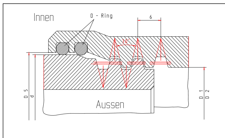
Skizze einer ABDI - Verbindung
